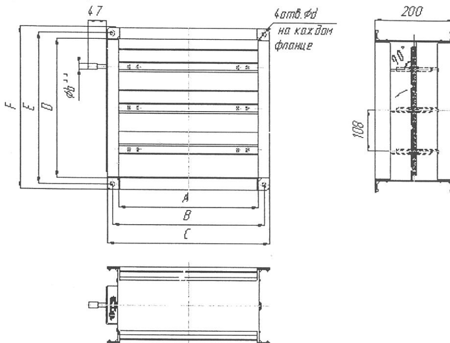
Рис.1 – габаритные, присоединительные и установочные размеры КВ.
